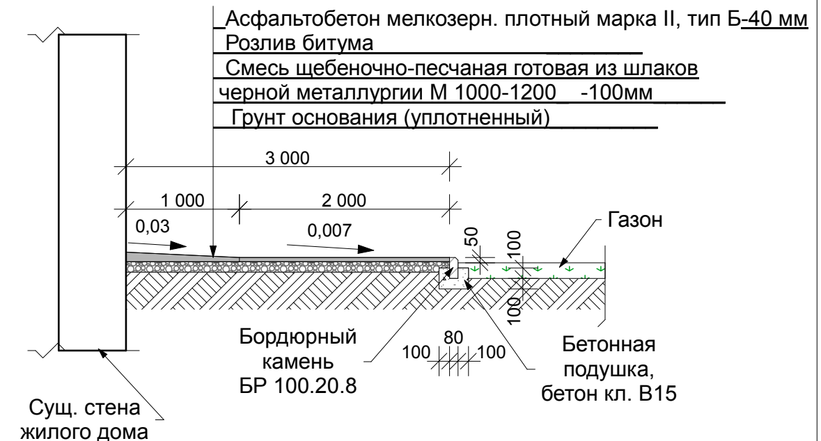
Сечение 2 - 2 (примыкание асфальтобетонного покрытия пешеходного тротуара к дому)
